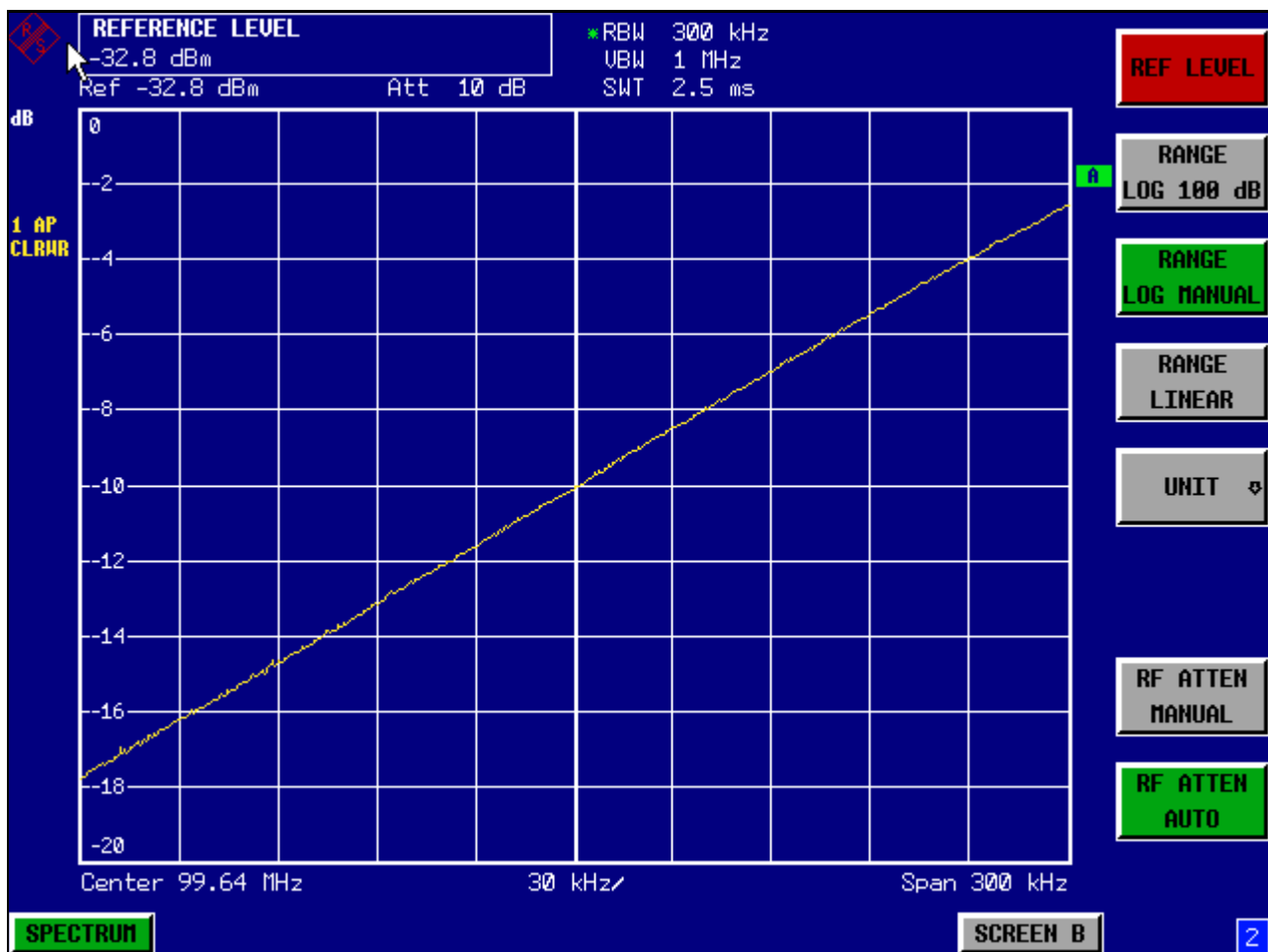
Fig. 5-14 Affichage du front d'un filtre 300 kHz utilisé comme caractéristique de discriminateur FM.
