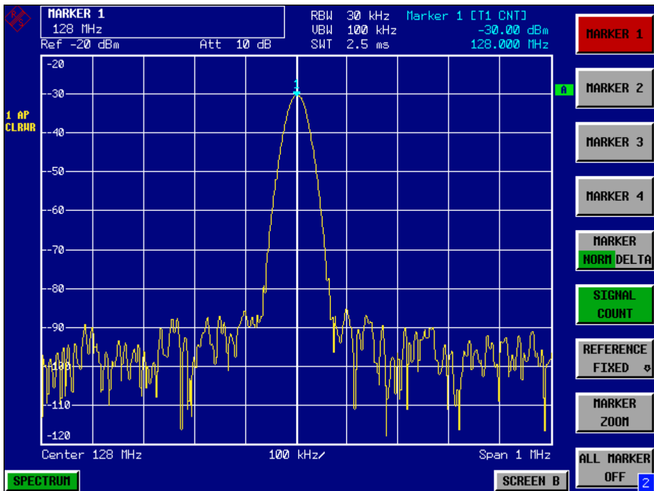
Fig. 5-1 Mesure de la fréquence à l'aide du compteur de fréquence
