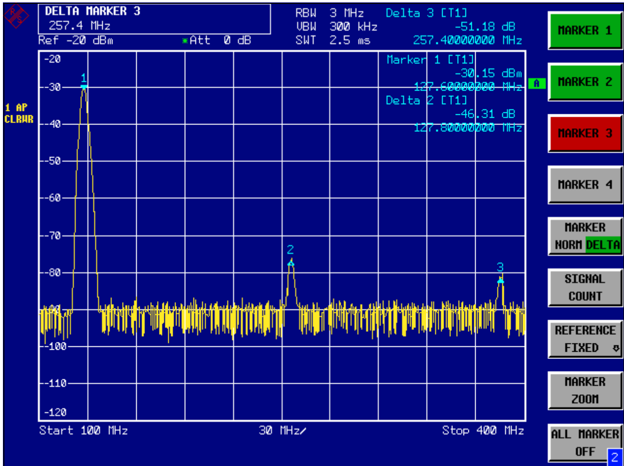
Fig. 5-2 Mesure de la réjection des harmoniques du générateur de référence interne. Les marqueurs delta 2 [T1] et delta 3 [T1] indiquent l'écart de la 1ère et de la 2ème harmoniques par rapport à la fondamentale.
