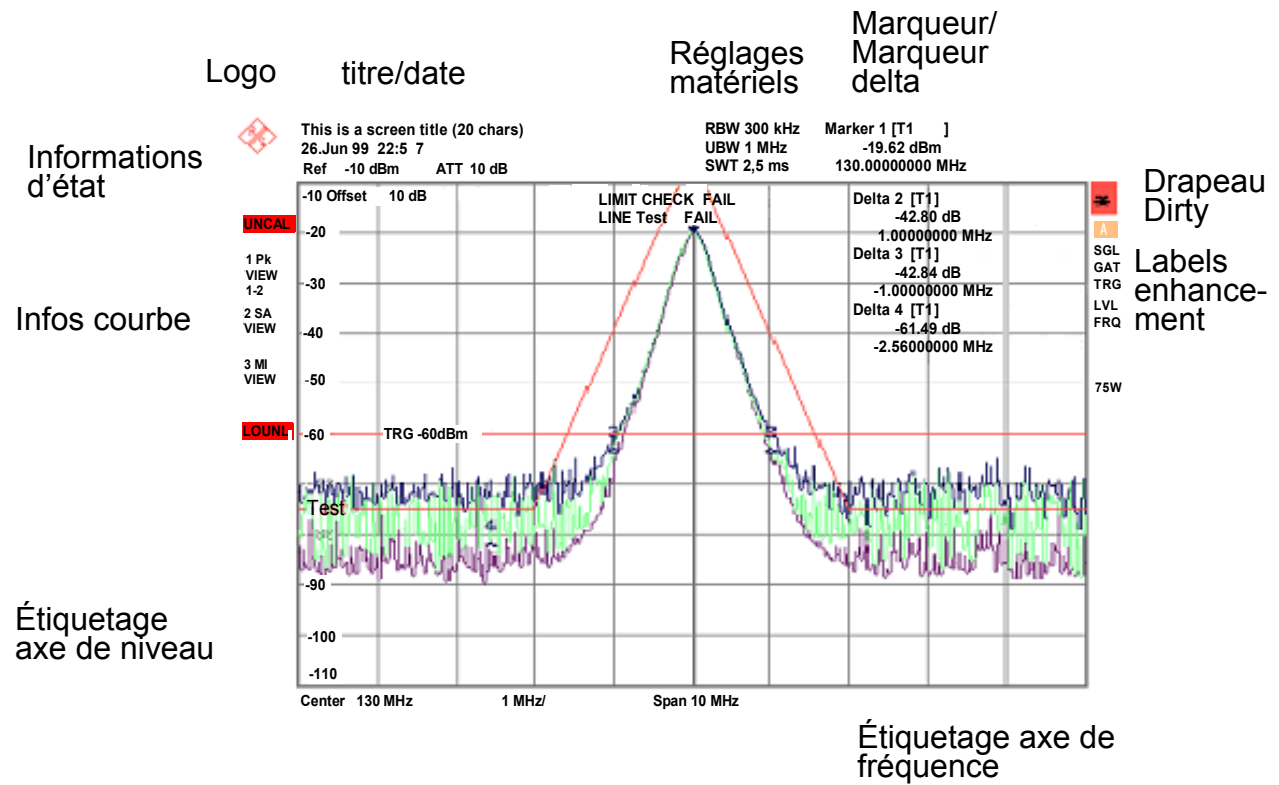
Fig. 4-1 Disposition de l'écran du R&S FSP en mode analyseur
