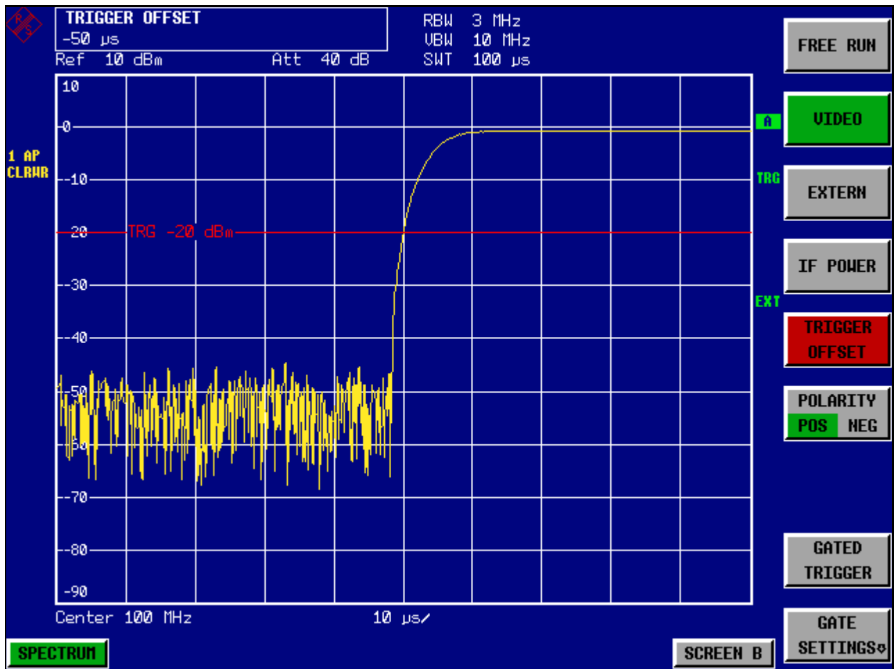
Fig. 5-9 Front ascendant du burst GSM à haute résolution temporelle.
