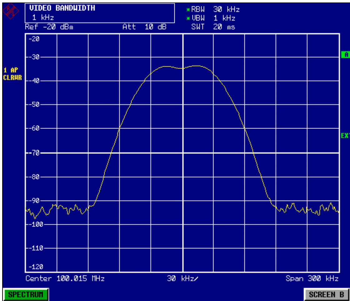
Fig. 5-4 Mesure de deux signaux RF sinusoïdaux égaux dont la largeur de bande de résolution correspond à l'écart de fréquence des signaux.
