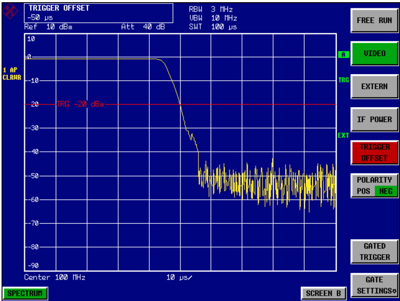
Fig. 5-10 Front descendant du burst GSM à haute résolution temporelle.
