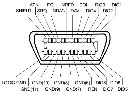
Fig. 1-9 Affectation des broches de la seconde interface CEI
