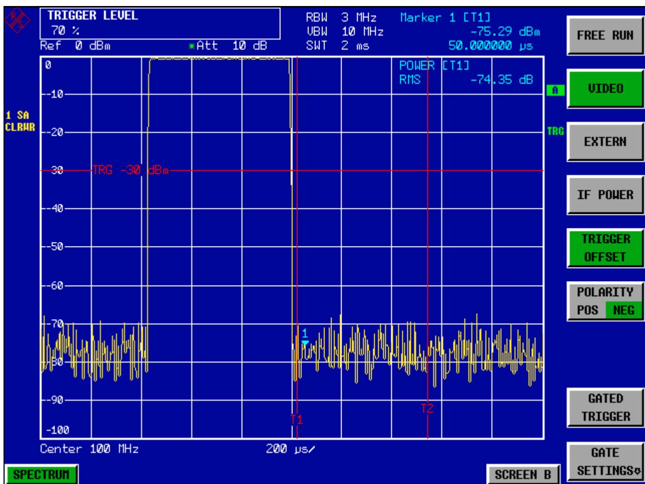
Fig. 5-12 Mesure du rapport signal/bruit d'un signal à bursts GSM dans le domaine temporel
