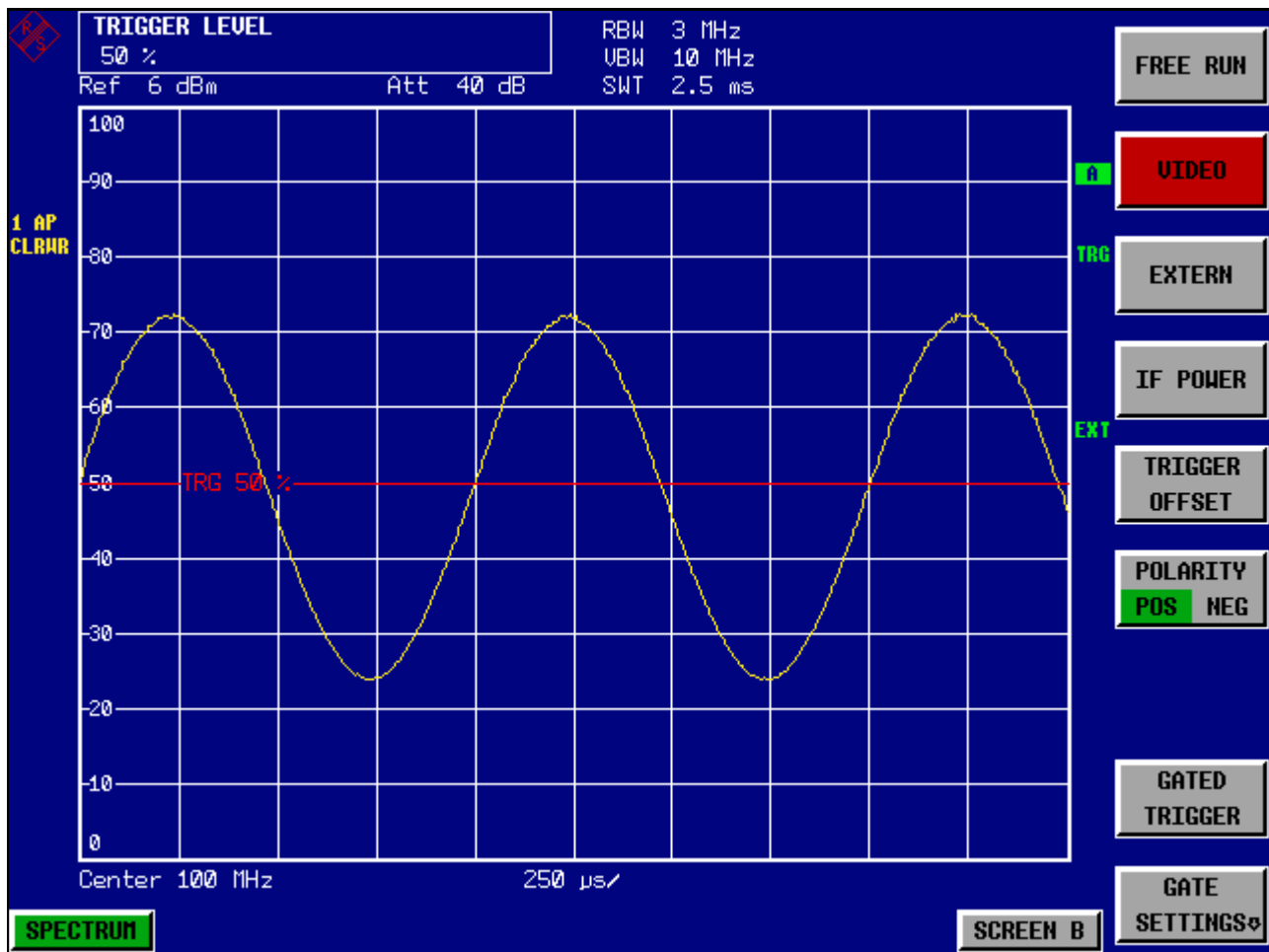
Fig. 5-13 Mesure du signal BF d'une porteuse de 1 kHz modulée en AM
