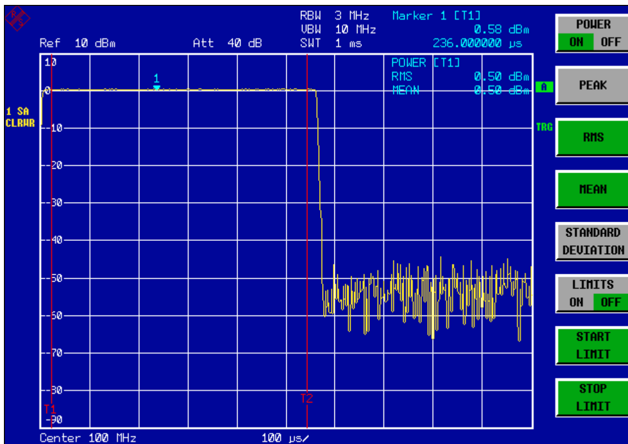
Fig. 5-8 Mesure de la puissance moyenne pendant la phase d'activation d'un burst GSM.
