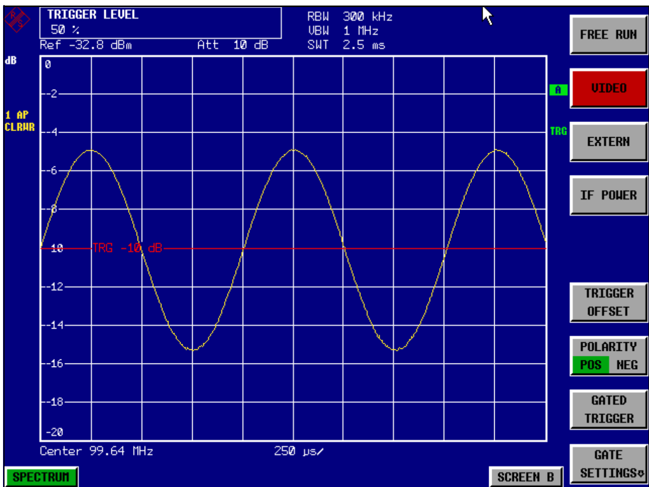
Fig. 5-15 Affichage du signal FM démodulé
